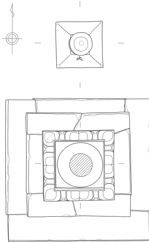
1 実測図（平面）
