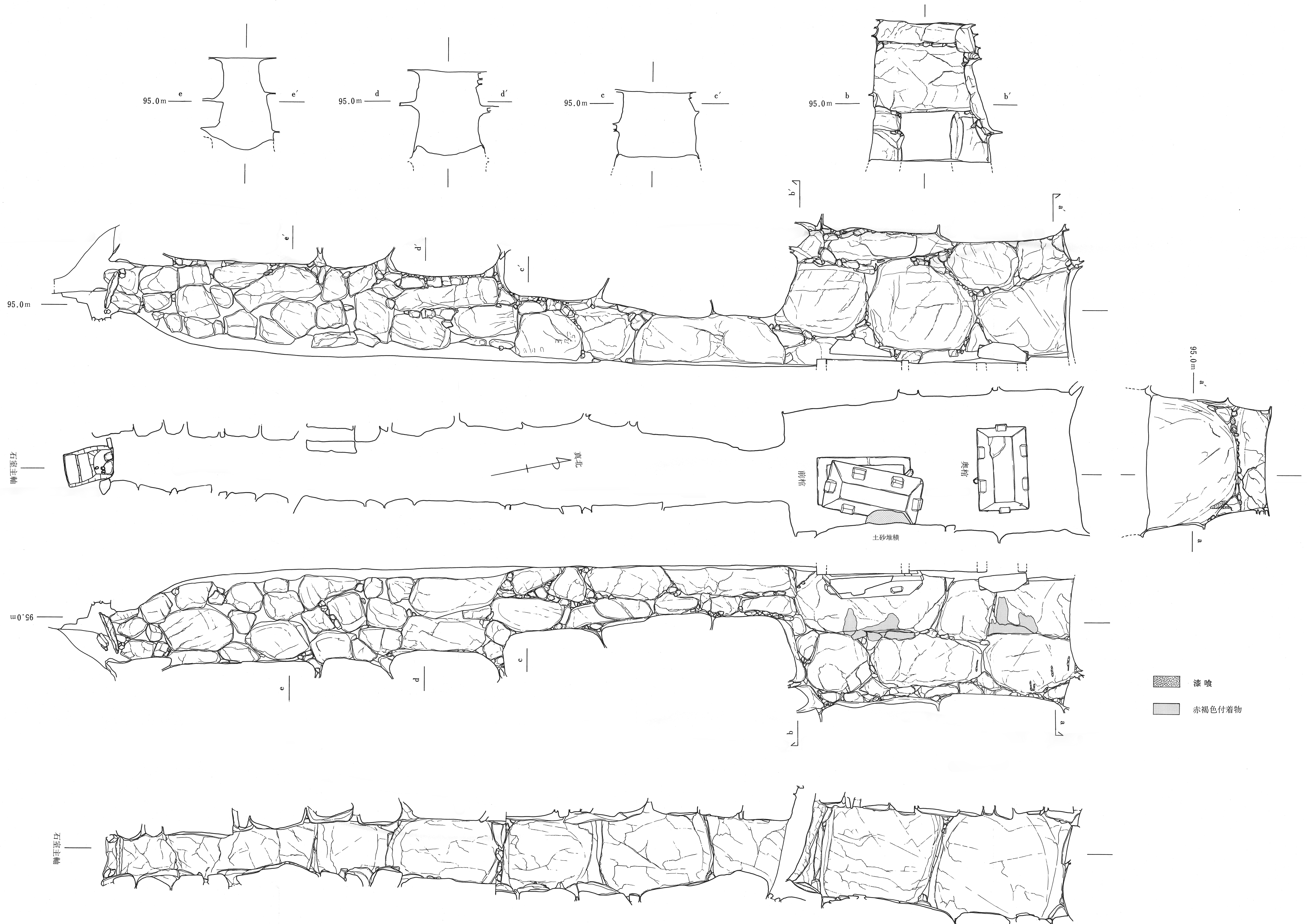
付図2 畝傍陵墓参考地横穴式石室実測図(1/50)
